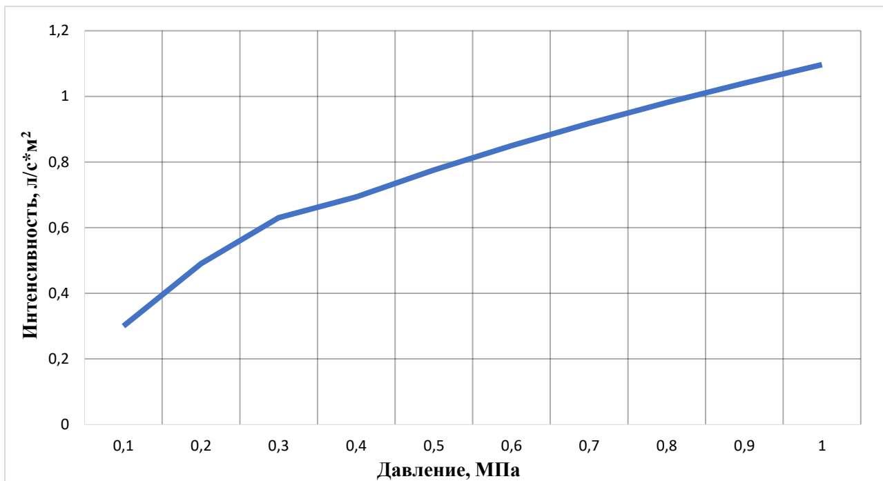
График зависимости интенсивности орошения от давления на площади 3 м 2
