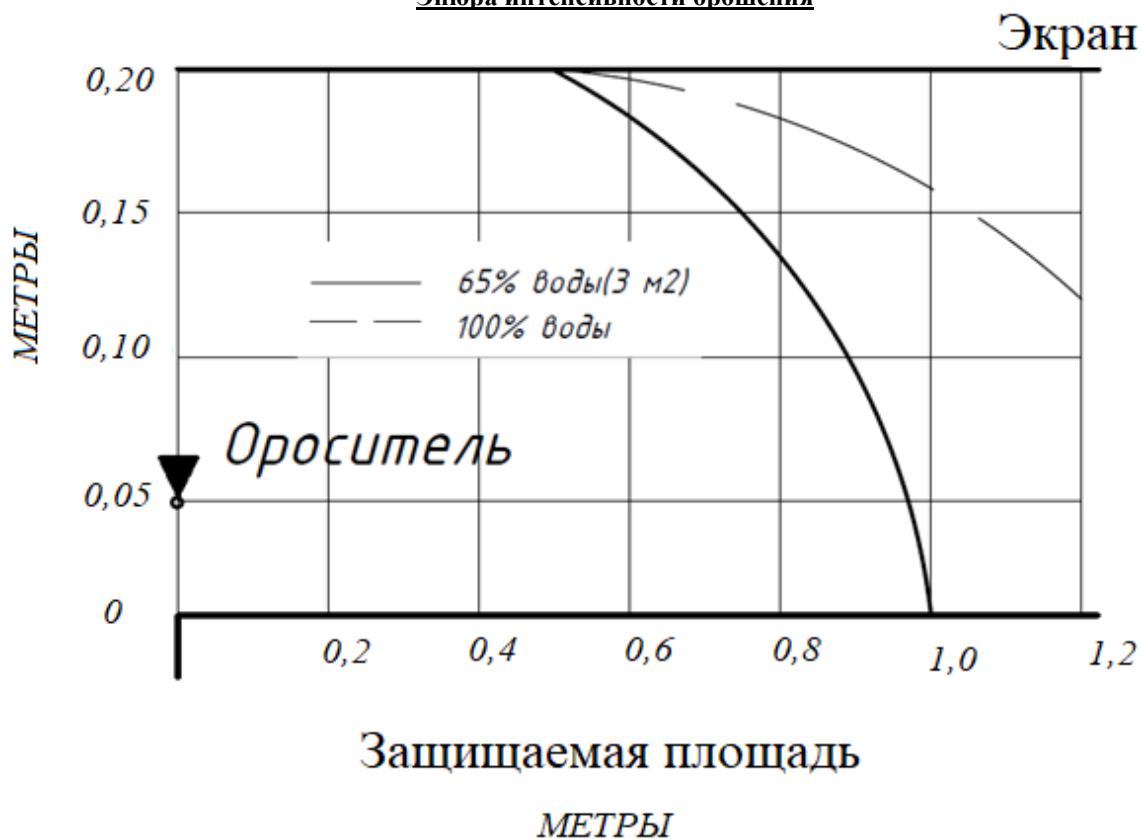
Эпора интенсивности орошения
